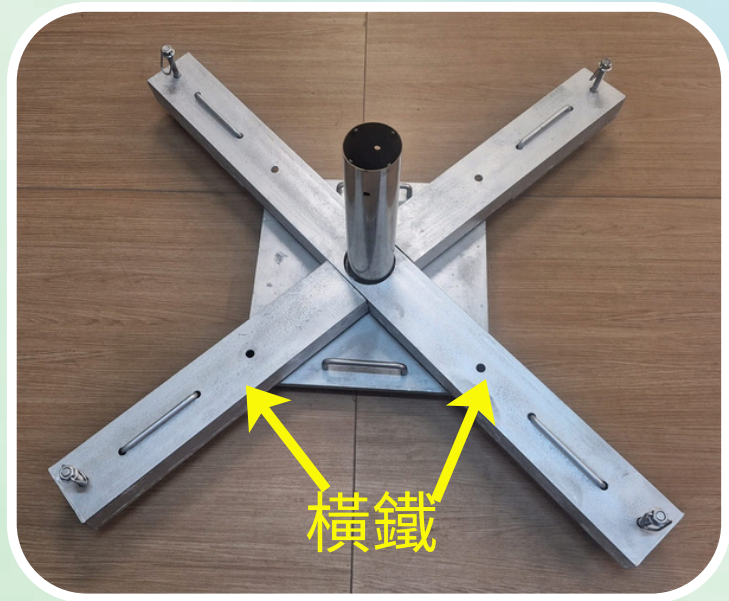
2. 底座：正方型的底座連橫鐵。
